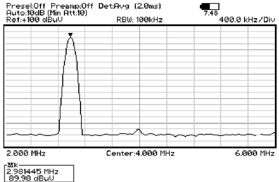
Fig. 15-3 Spectrum
