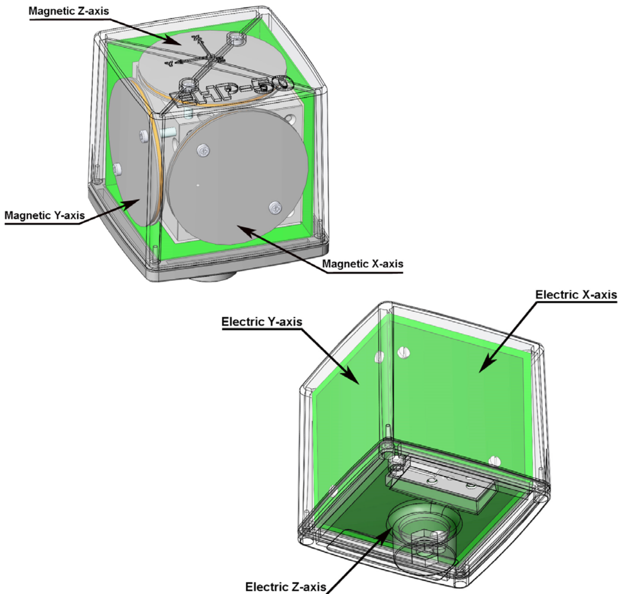
Fig. 1-3 EHP-50G axes
